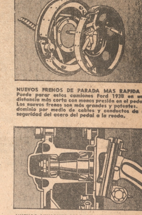
NUEVOS FRENOS DE PARADA MAS RAPIDA - Puede parar estos camiones Ford 1938 en una distancia más corta con menos presión en el pedal. Los nuevos frenos son más grandes y potentes. El dominio por medio de cables y conductos de seguridad del acero del pedal a la rueda.
