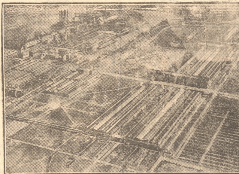
VISTA AEREA DE LA PLANTA FORD MOTOR COMPANY EN RIO ROUGE DEARBORN, MICHIGAN, E. U. A. CUBRE UNA EXTENSION DE 443 HECTAREAS
