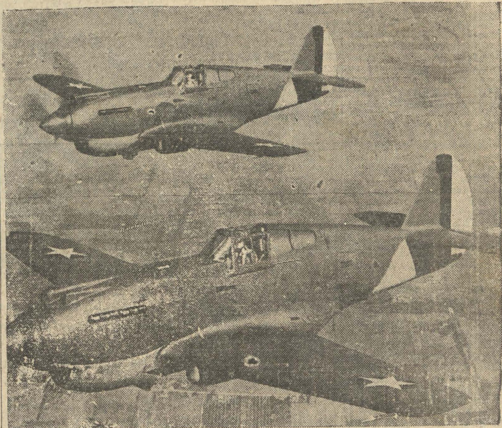
Dos de los aviones de combate Curtiss P-40 del ejército norteamericano, volando sobre Buffalo, Nueva York. Diseñados para combates a grandes alturas, son de un solo pasajero e iguales a los aviones de combate construidos por Curtis para la Real Fuerza Aérea británica (Foto de la I. I. News.)
