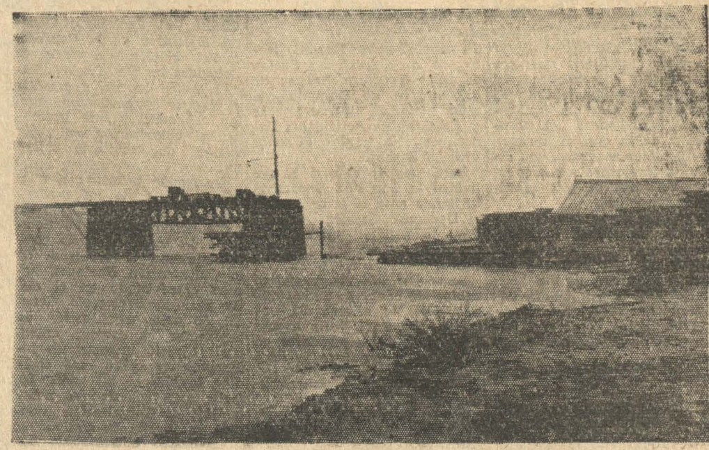
La crecida del Bio-Bio llegó a uno de sus puntos más altos en esta parte en que están afirmando los primeros pilares del futuro puente carretero
