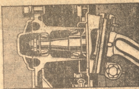
NUEVOS MUNONES MAS GRANDES — Un factor aumentado de seguridad para los camiones de 285 cms. y 399 cms. lo suplen munones más grandes con pernos de mayor tamaño. La superficie más grande de los pernos y bujes reduce el desgaste. El nuevo diseño del munón mejora la acción del conductor.
