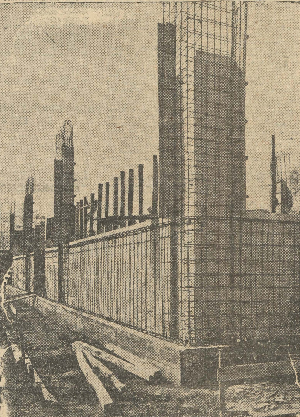
Este enfierramiento corresponde a nuevos pabellones que se alzarán en los terrenos adyacentes a la moderna Fábrica de Radios RCA Victor, con motivo de su plan de extensión. Aquí será donde otro centenar de brazos chilenos trabajarán para el engrandecimiento y prosperidad de la industria nacional.
