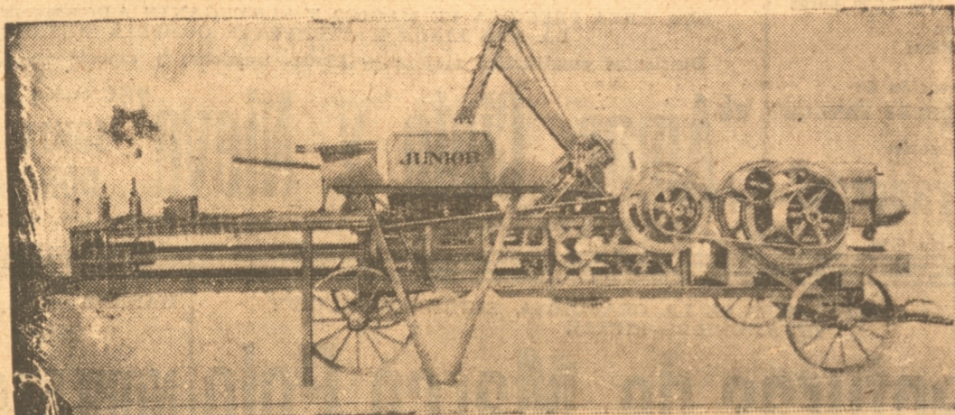
Prensa para Pasto a Motor
