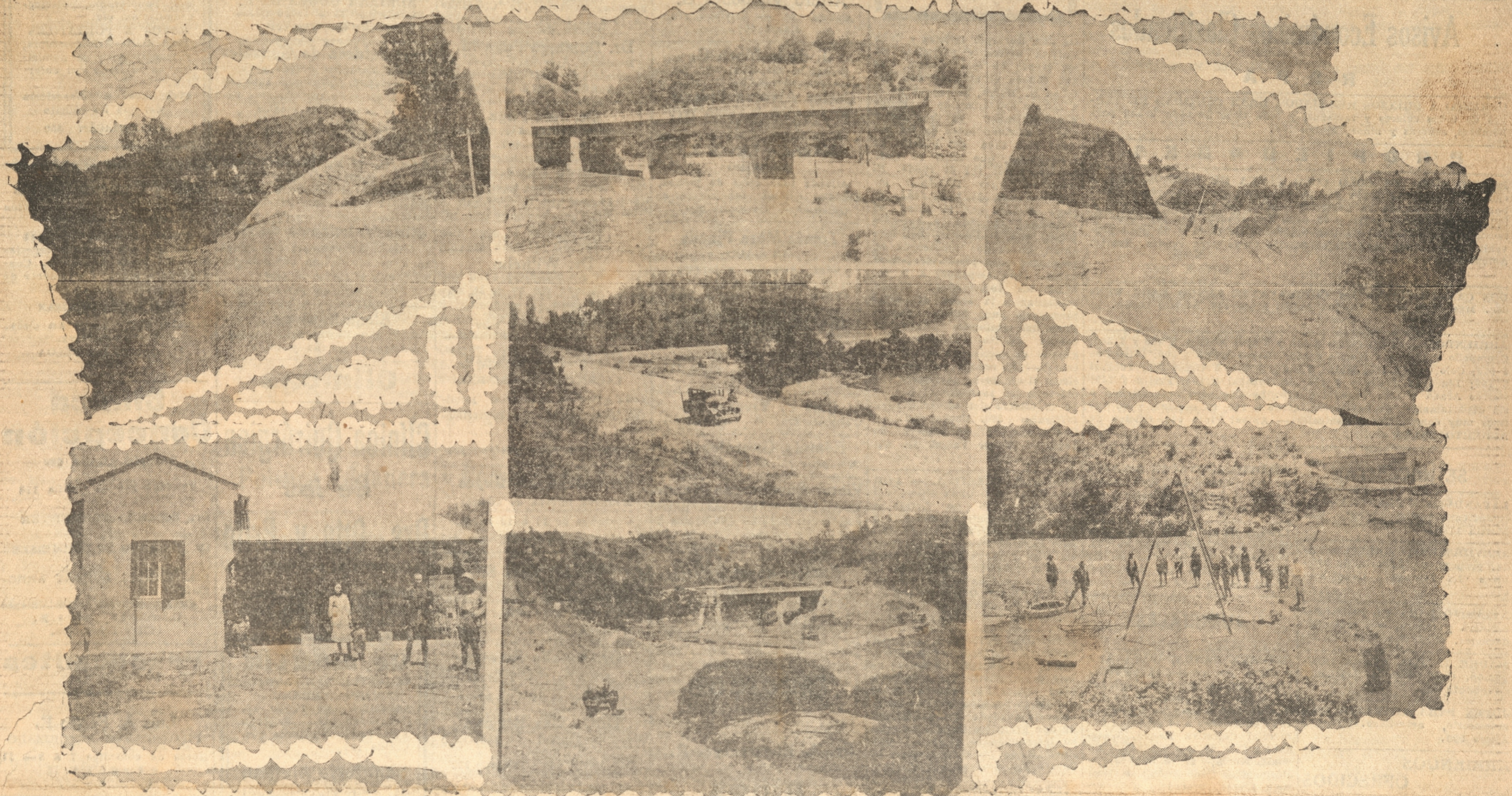
1).—TERRAPLEN DEL CORTE DE LOS CARACULES (kilómetro 4).— 2).— PUENTE NUMERO 1 SOBRE EL RIO ANDALIEN, QUE ESTA TERMINADO.— 3).— PERSONAL DE LA INSPECCION TECNICA, TRABAJANDO EN EL KILOMETRO 26.— 4).— UNA INTERESANTE PERSPECTIVA DEL CAMINO, EN EL KILOMETRO 17.— 5).— CASA DE CAMINERO EN EL KILOMETRO 26.— 6).— PUENTE NUMERO 4, EN CONSTRUCCION.— 7).— EL INGENIERO SEÑOR LATHAM TRABAJANDO EN UNA DE LAS EXCAVACIONES DEL PUENTE NOR 5, EN CONSTRUCCION.
