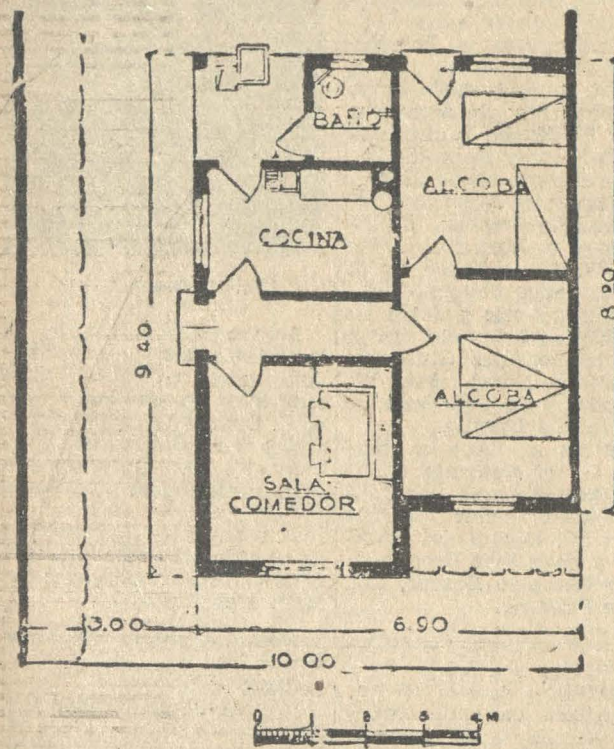
Un plano modelo para casas económicas elaborado por el Departamento de Urbanismo de Bogotá.
