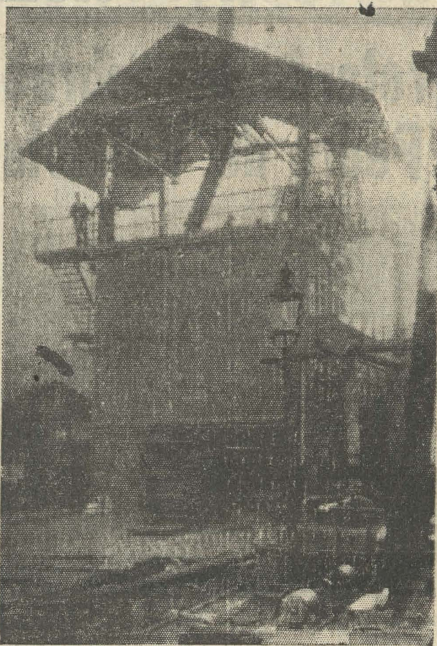
Una vista de la nueva planta inaugurada ayer. El carro que está casi a la entrada llevará el coque a la torre de apagamiento.
