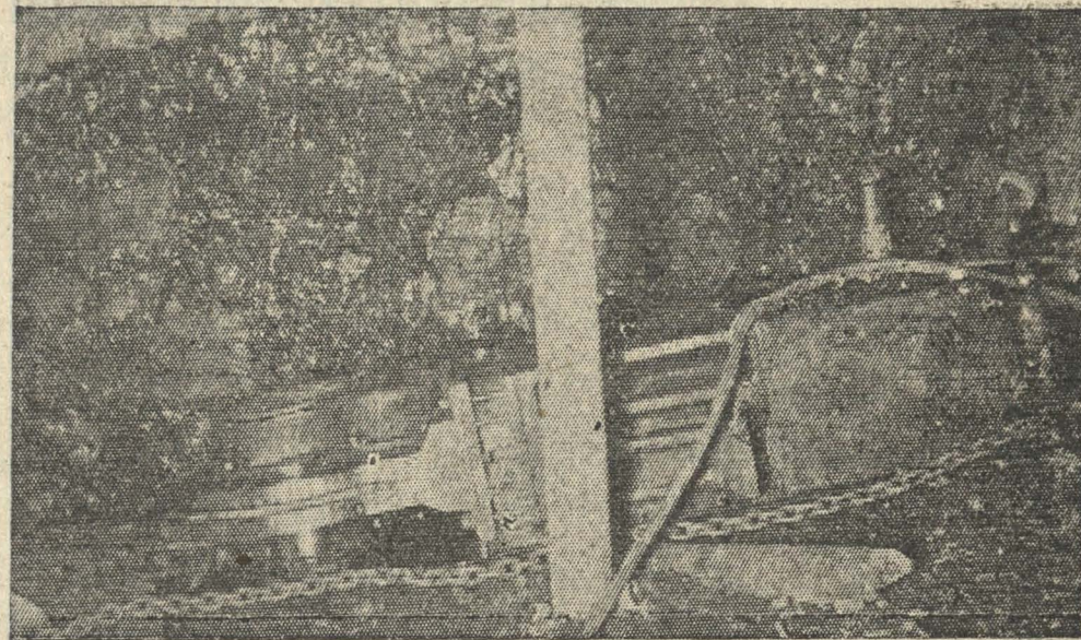
CIRCADORA EN TRABAJO EN EL INTERIOR DE LAS MINAS DE LOTA
