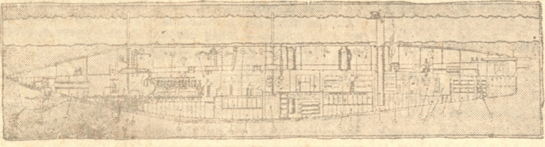
Corte longitudinal del "Nautilus" que muestra las distintas reparticiones, después de los arreglos a Sir Hubert Wilkins y su esposa La dy Wilkins que le acompañará en su expedición a las regiones árticas
