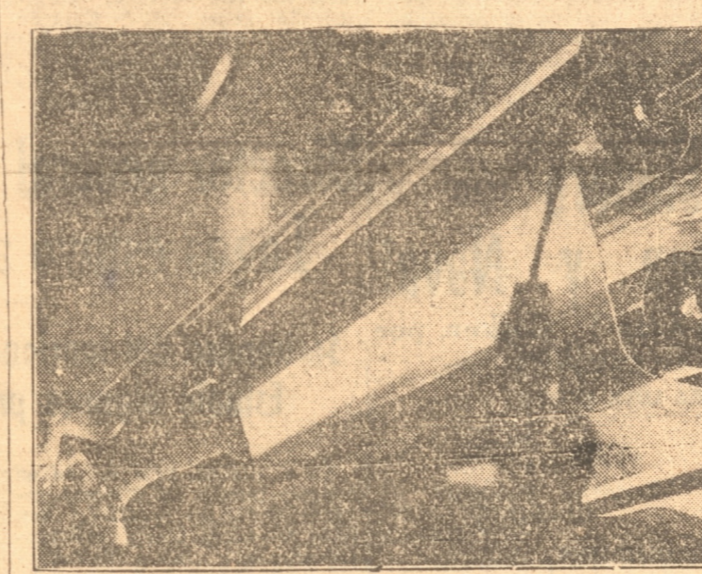
En el granadero se ve la película de celulosa saliendo del baño de coagulación, en el cual se transforma en rápida marcha en la fábrica de clar-apel en Richmond, Virginia
