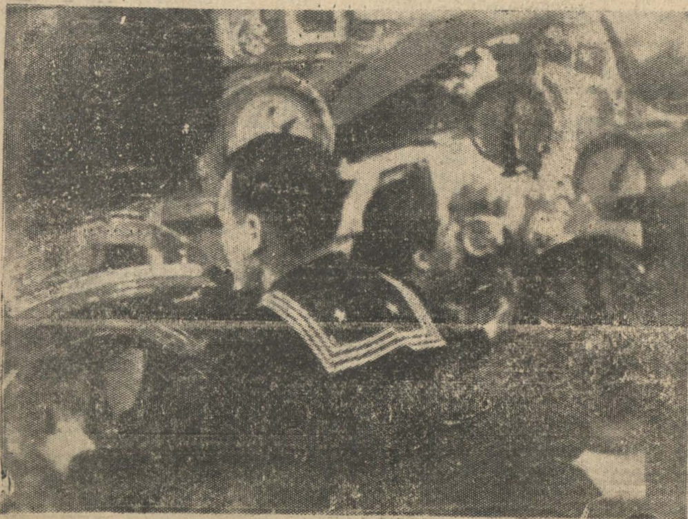
En esta sección se lleva el control de profundidad del submarino.— Fué tomada en el "Thompson".— Aparecen dos de los timoneles, personal especializado de gran competencia.
