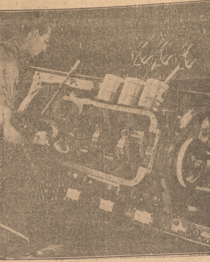
Cada una de las piezas que integran los motores Diesel es objeto de prolongada y minuciosa inspección en las fábricas de la International Harvester.
