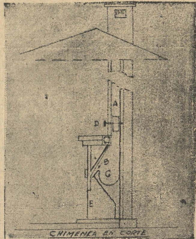
A) Tubo de humo, B) paso de salida, C) Cámara de humo, D) Templador, E) Boca o abertura.
